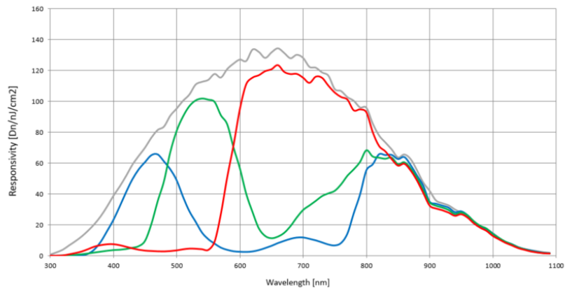
预测的光谱响应率红绿蓝+单色
